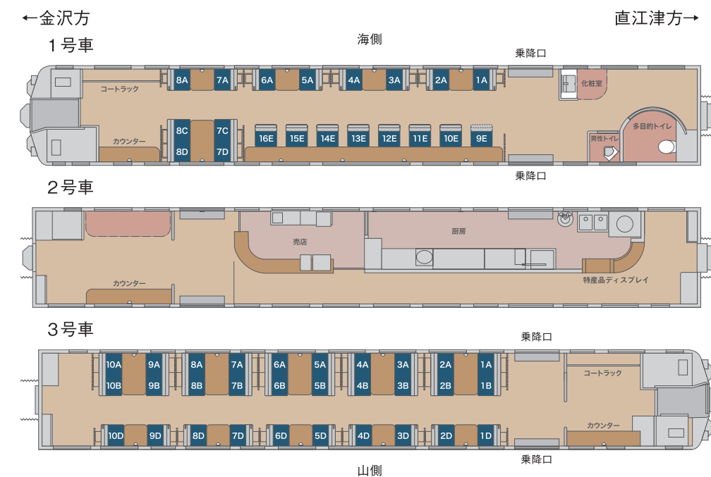
客席 (1・3号車)
